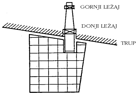
VISEĆE KORMILO
